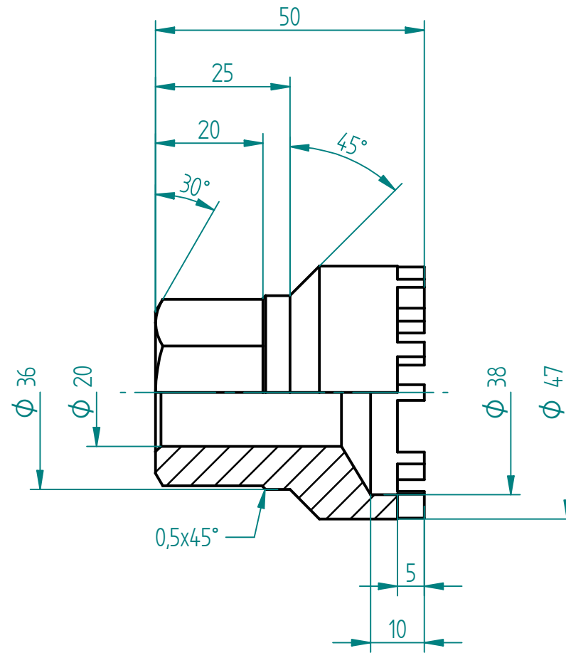
SCHNITT A-A
