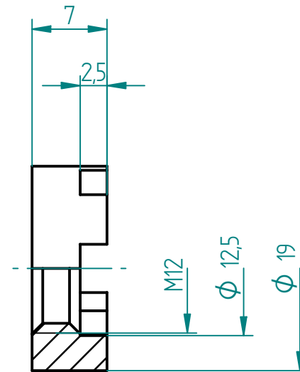
SCHNITT A-A
