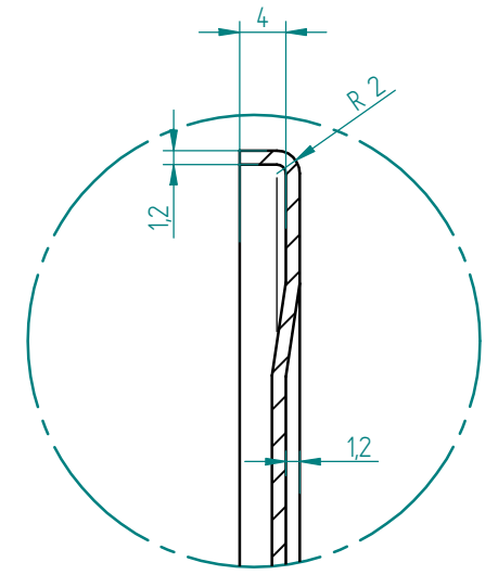
EINZELHEIT B
